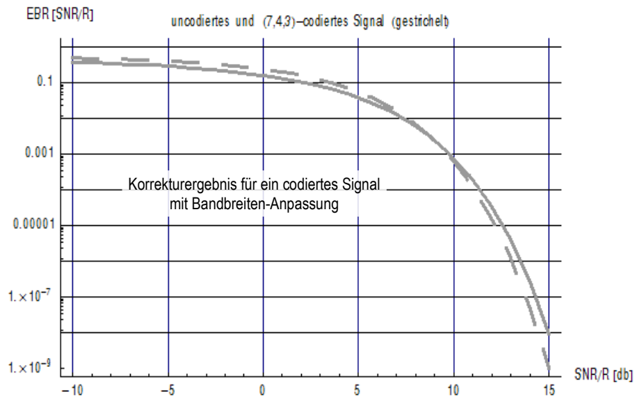
Mittlere Fehlerverläufe für ein uncodiertes Signal (durchgezogene Linie, wie in Bild 3.3) und ein Hamming-codiertes Signal bei gleicher Übertragungsgeschwindigkeit der Info-Bits
